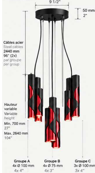
VUE DE FACE FRONT VIEW
